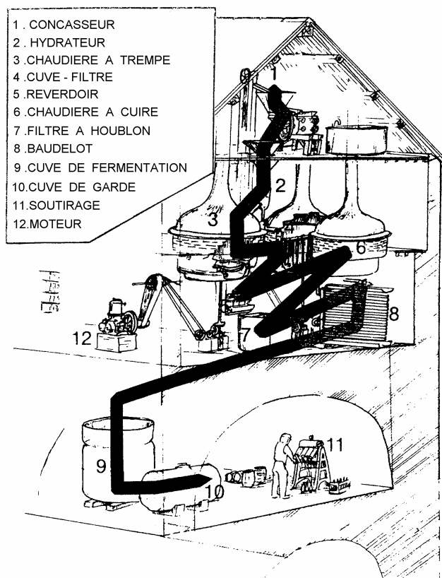
LA FABRICATION DE LA BIÈRE AU MUSÉE DE LA BIÈRE DE STENAY - MATÉRIEL DE CLAVY-WARBY (08)
