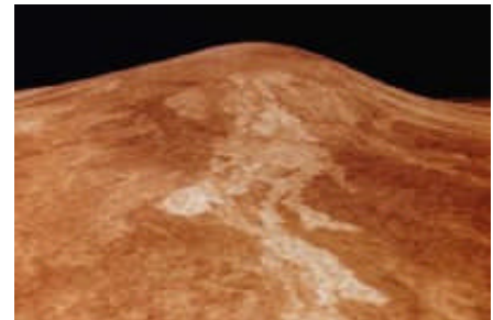
Le volcan Sif Mons à la surface de Vénus dont les coulées de lave témoignent d'une activité passée. Image de la sonde Magellan (NASA)
